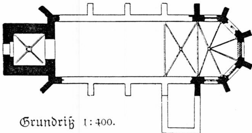
Grundriß der Kirche St. Paulus zu Hervest bis 1895 ( entnommen aus : BKW Landkreis Recklinghausen , a.a.O., S. 281.)
